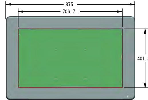
Transparent Liquid Crystal Display Show Box / 透過型液晶ディスプレイショーボックス
